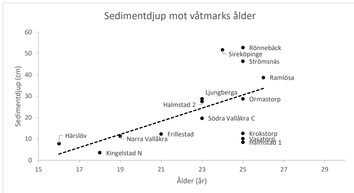
Figur 9. Genomsnittligt sedimentdjup i våtmarken i relation till våtmarkens ålder. Streckad linjär trendlinje där R^2 = 0,307 ; p = 0,033 .
