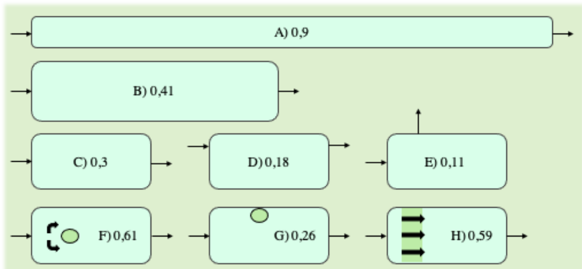
Figur 3. Exempel på värden på hydrauliska effektiviteten beroende på våtmarksutformning. Bilderna är numrerade från A-H. Inlopp och utlopp markeras med pilar. I våtmark F och H markeras även vattnets flödesväg med grövre pilar i våtmarkerna. Gröna cirklar i våtmark F och G symboliserar öar. Gröna området, vertikalt mot flödesvägen, i våtmark H symboliserar en växtbank som hjälper till att sprida vattnet. Illustration: Louise Lumsén baserad på (Persson 2000).
